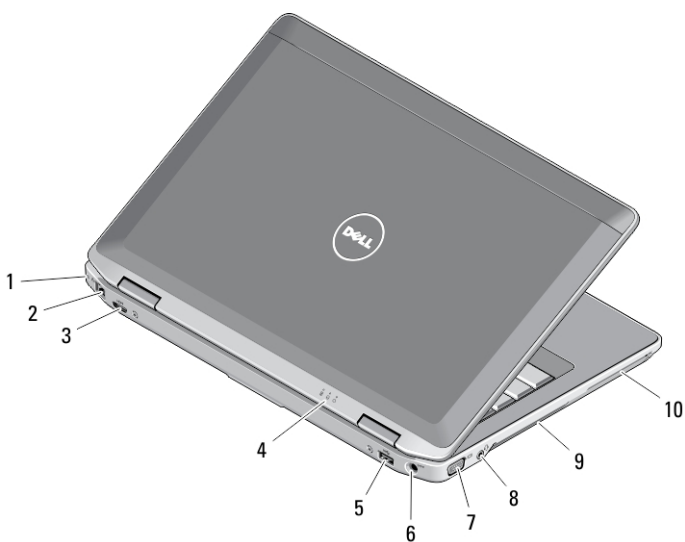
Figur 2. Sett bakfra
